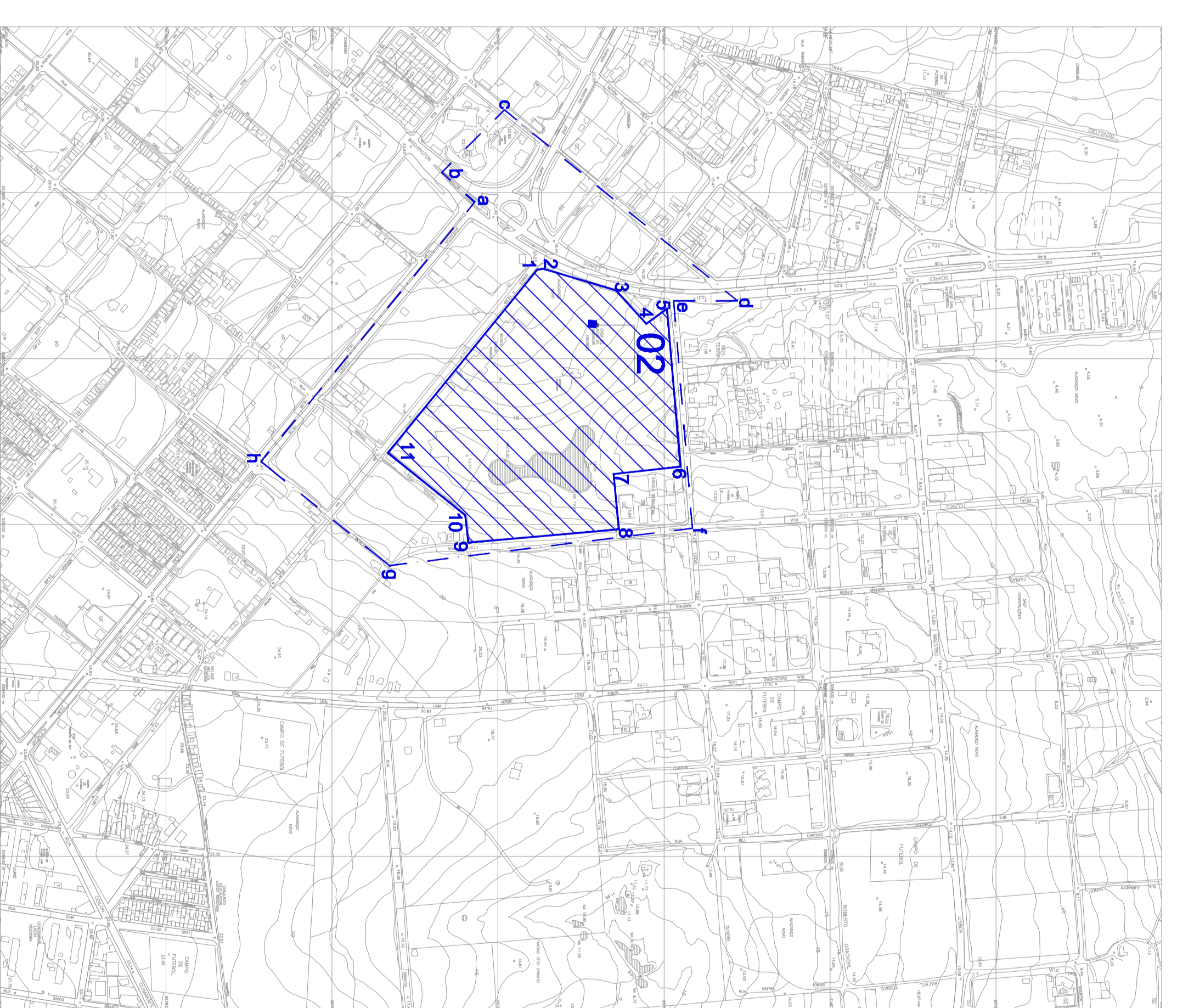
3 DETALHE 3 DA PLANTA DA REGIONAL VI DE FORTALEZA ESCALA 1/5000
