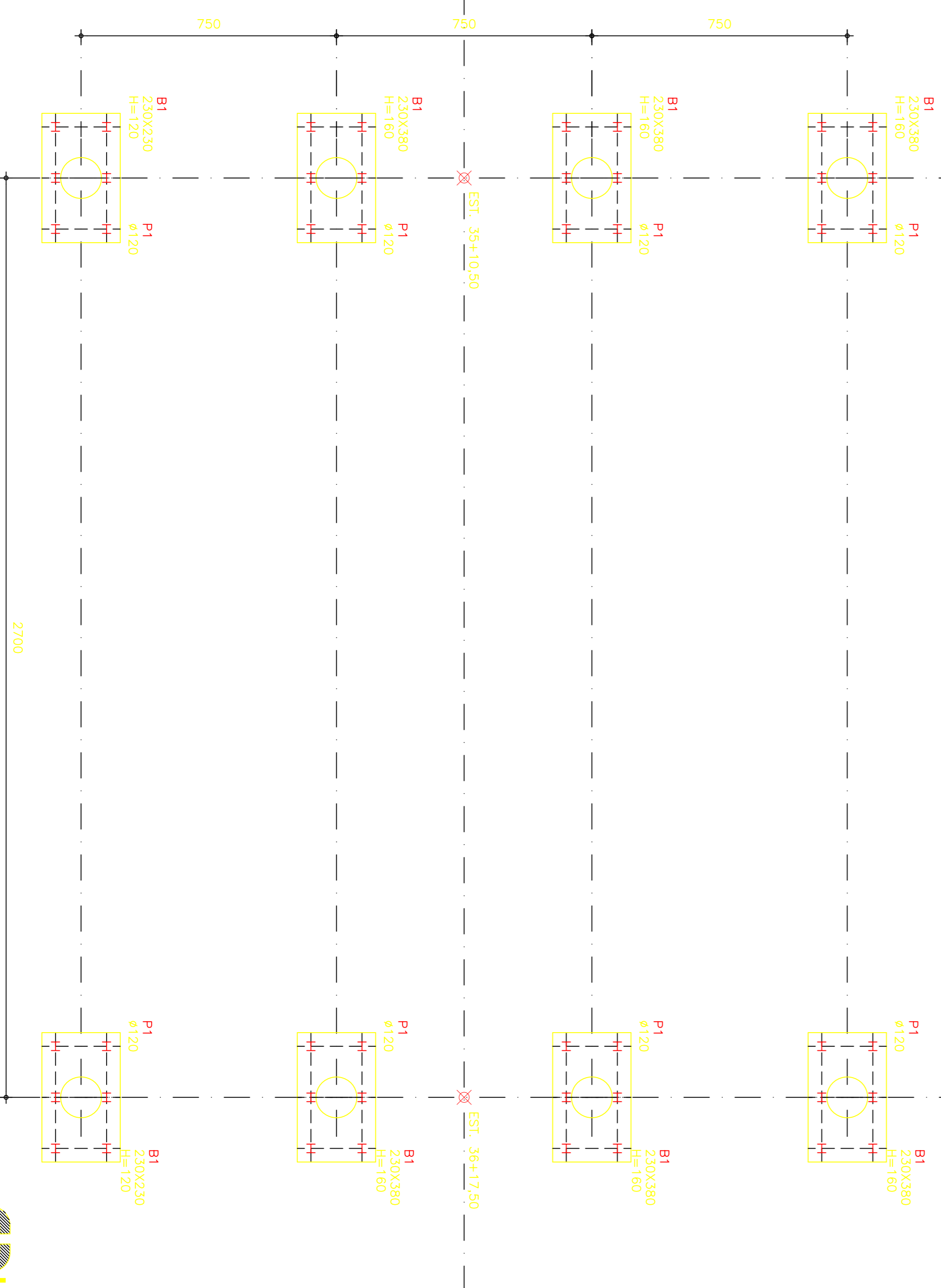
LOCAÇÃO DAS FUNDAÇÕES ESCALA 1:100
