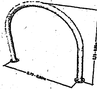
Figura 1 - Modelo - Paraciclo
