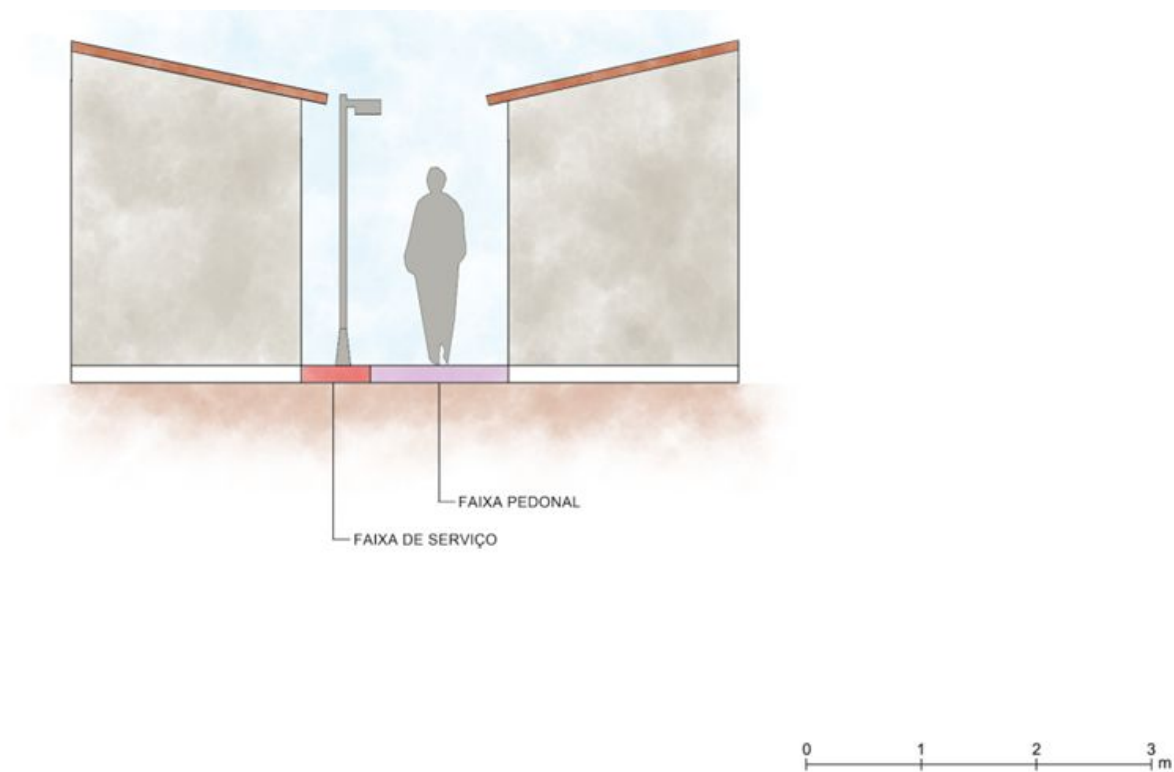
Figura 02: Corte esquemático da via pedonal tipo B. Fonte: Equipe técnica UNIFOR, 2019. Elaboração: Equipe Técnica UNIFOR.
