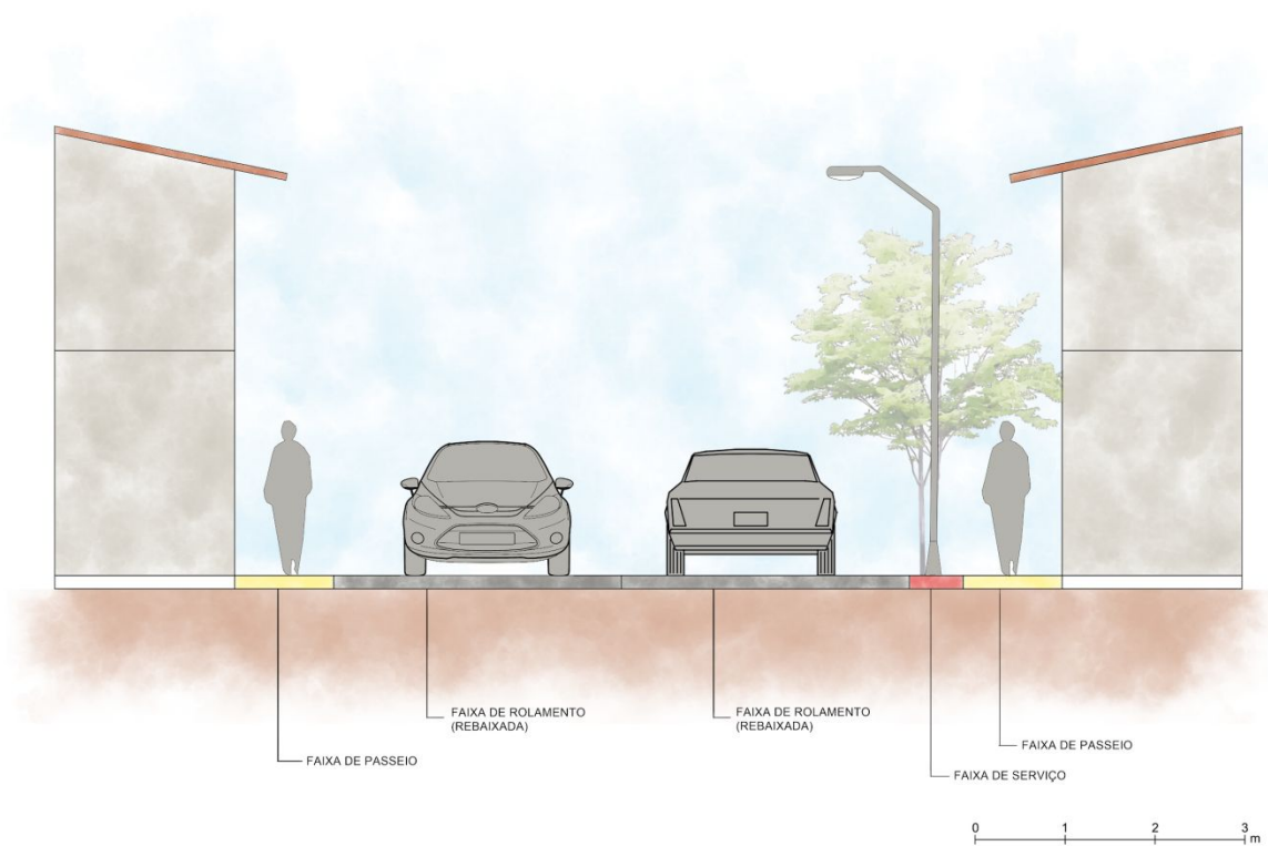
Figura 02: Corte esquemático da via local especial tipo B. Fonte: Equipe técnica UNIFOR, 2019. Elaboração: Equipe Técnica UNIFOR.
