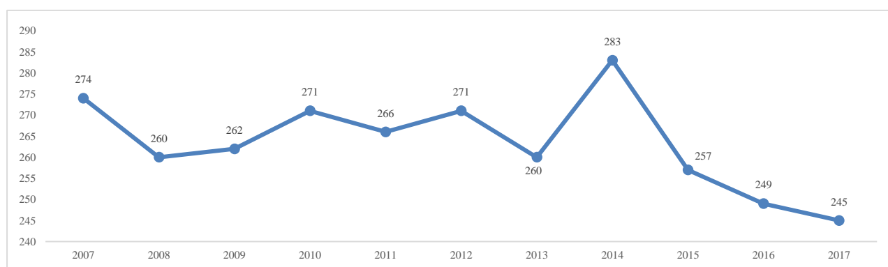
Gráfico 5: Evolução do número de aeroportos de destino das decolagens aéreas com origem no Brasil - 2007 a 2017
