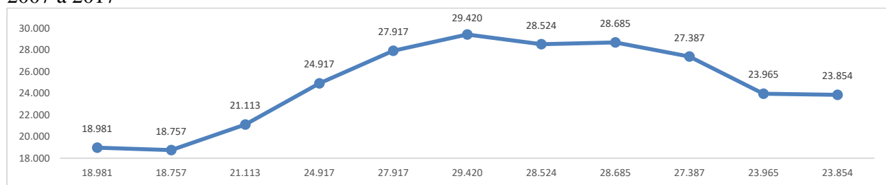
Gráfico 17: Evolução do número de decolagens aéreas que tem como origem o estado do Ceará - 2007 a 2017
